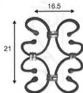
INSERT # 6 ESPECIAL P086
