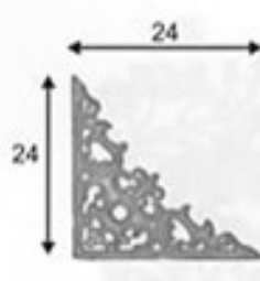
ESQUINERO CHICO 3 P721
