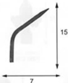
PUNTA DOBLADA P087 C 1/2" P092 C 3/8"
